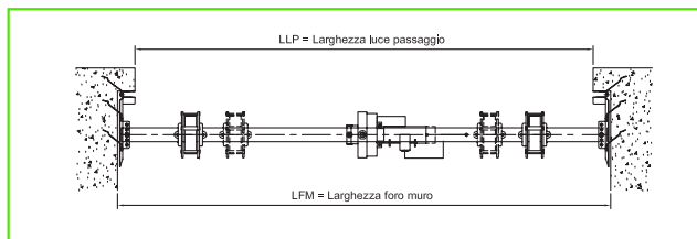
Sezione orizzontale
