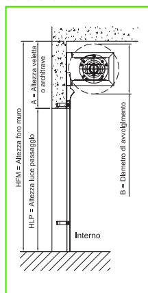
Sezione verticale
