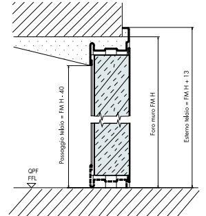
Sezione verticale REI 60 / REI 120
